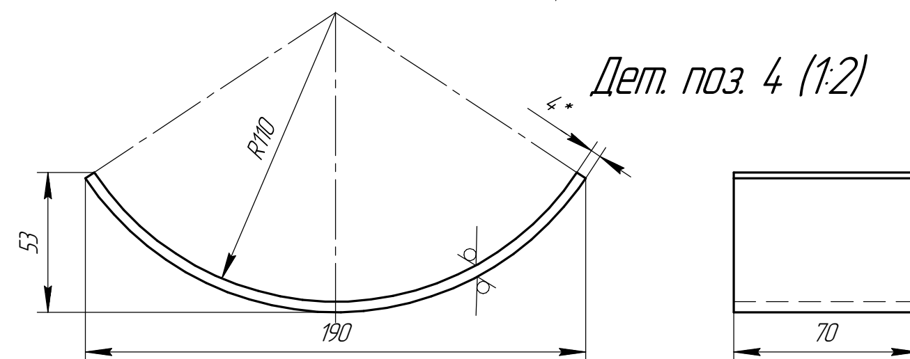
Det. poz. 4 (1:2)
