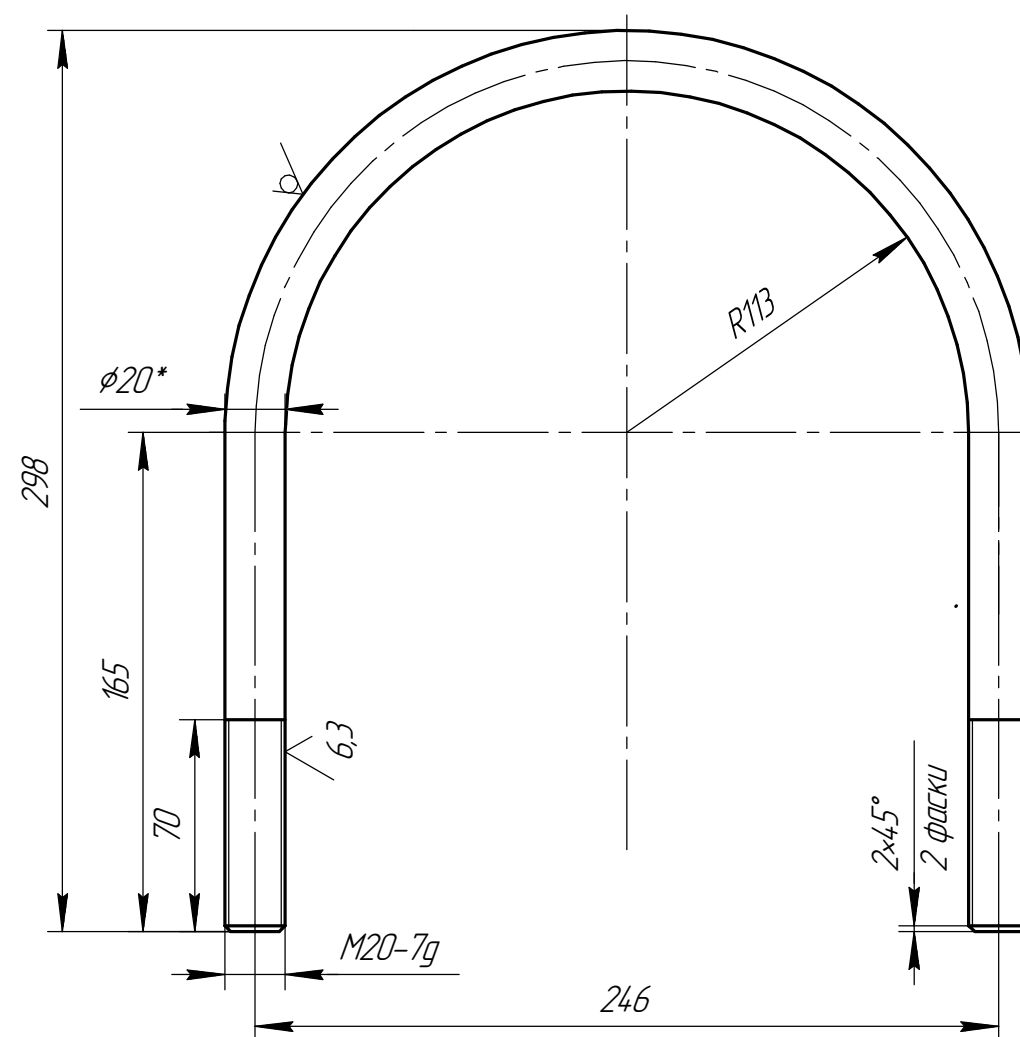
Det. poz. 4 (1:2)
