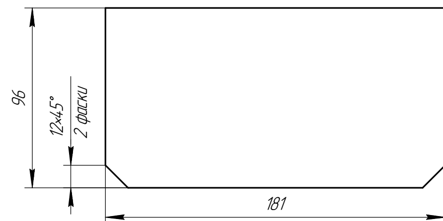
Det. poz. 2 (1:2)
